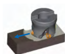
Фрезерование плоскости
