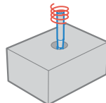
Фрезерование по винтовой интерполяции
