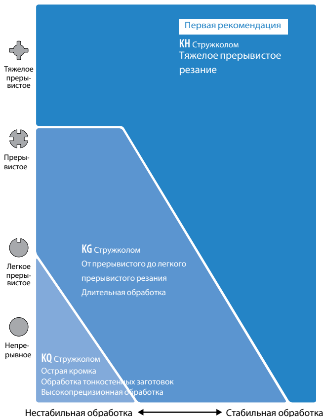
Recommended K-Series chipbreakers
